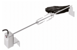
Quasar Rotisserie-Set bestehend aus: 1 Drehspieß, 2 Edelstahl Fleischklammern, 2 spezielle Halterungen zur Montage, 1 Motor 230V, 1 Paar Schutzhandschuhe
